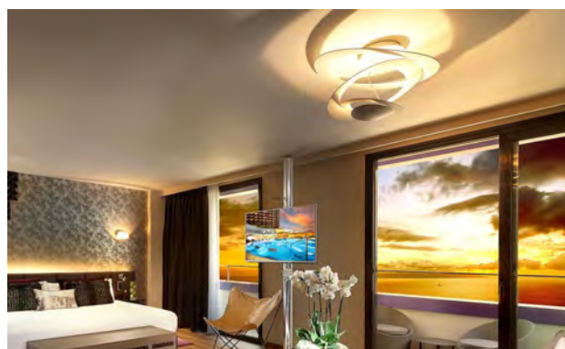
PIRCE MINI SUSPENSION LED WHITE/GOLD ¥308,000(税抜 280,000円) ・内臓LED 44W 3000K 3313lm ・W:670 D:690 H:230 全長:max2000 4.6kg ・アルミ塗装仕上
