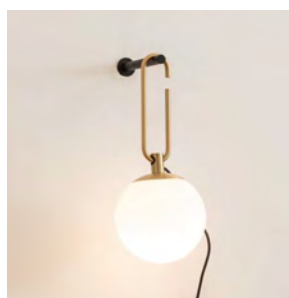
nh WALL ¥79,200(税抜 72,000円) ・E17 LED電球 40W型 電球色 x1 ・W:140 D:197 H:326 1.0kg ・ガラス、真鍮、鋼 ・コンセント用プラグ付き
