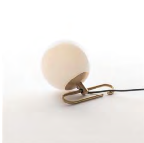
nh 1217 TABLE ¥77,000(税抜 70,000円) ・E17 LED電球ホワイト 40W型 電球色 x1 ・W:170 D:140 H:204-324 0.9Kg ・ガラス、真鍮 ・中間ON-OFFスイッチ付
