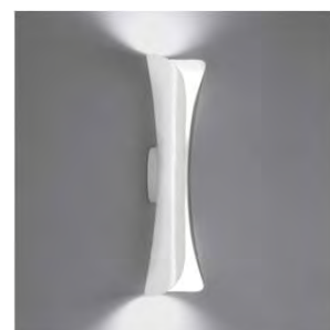
CADMO WALL LED WHITE ¥143,000(税抜 130,000円) ・GU10 LED電球(電球色) 7.5W X2 ・W:131 D:134 H:540 1.2kg ・アルミ、樹脂
