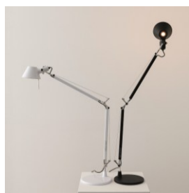
TOLOMEO TABLE (BLACK/WHITE) ¥90,200(税抜 82,000円) ・E17 ミニクリプトランプホワイト60Wx1 ・W:780-1220 D:230 H:645-1290 4.7kg ・アルミ塗装仕上 ・スイッチ付
