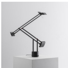
TIZIO BLACK ¥104,500(税抜 95,000円) ・GY6.35 ハロゲンランプ(低内圧型) 12V50W x1 ・W:110-1090 D:110 H:320-1180 3.5kg ・鋼塗装仕上、プラスチック ・調光スイッチ付(100%-50%-OFF)
