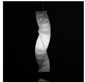
IN-EI TATSUNO-OTOSHIGO ¥352,000(税抜 320,000円) ・内臓LED29W 3000K 2119lm ・W:386 D:386 H:1500 全長:2700 2.9kg ・鋼、樹脂 ・LED電源別置
