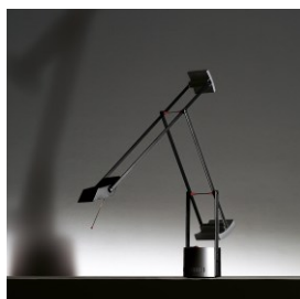
TIZIO MICRO BLACK ¥82,500(税抜 75,000円) ・G4 ハロゲンランプ(低内圧型) 12V20W x1 ・W:86-679 D:86 H:228-761 1.8kg ・鋼塗装仕上、プラスチック ・調光スイッチ付(100%-50%-OFF)
