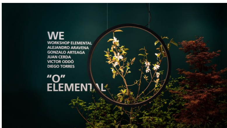
“O”45 OUTDOOR ¥242,000(税抜 220,000円) ・内臓LED 19W 3000K 875lm ・W:472 D:100 H:460 3.0kg ・アルミ塗装仕上、ステンレス ・防雨型:IP67
