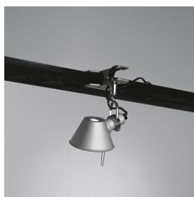
TOLOMEO MICRO PINZA ¥41,800(税抜 38,000円) ・E17 ミニクリプトンランプ 40Wx1 ・W:160 D:110 H:max275 0.4kg ・アルミアルマイト仕上 ・中間スイッチ付 コンセント付 ・対応板厚18-30mm ・照射面近接限度0.2m
