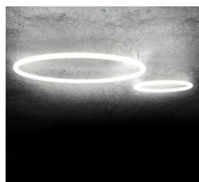
ALPHABET OF LIGHT CIRCULAR 90 ¥440,000(税抜400,000円) ・内臓LED 56W 3000K 6041lm ・W: φ900 H:50 全長:500-1500 6.5kg ・樹脂、銅 ・電源別置
