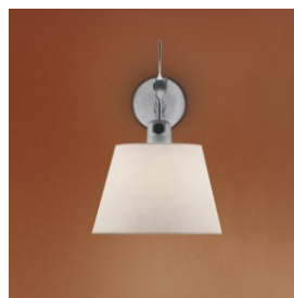
TOLOMEO DIFFUSORE 24 WALL (PARCHMENT/GREYSATIN) ¥104,500(税抜 95,000円) ・E26 LED電球ホワイト 60W型 電球色 ・W:368 D:240 H:352 0.7kg ・アルミアルマイト仕上 ・セード:パーチメント(紙) or グレイサテン(布) ・スイッチ付
